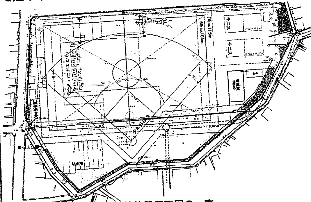
競技施設平面図の一案
