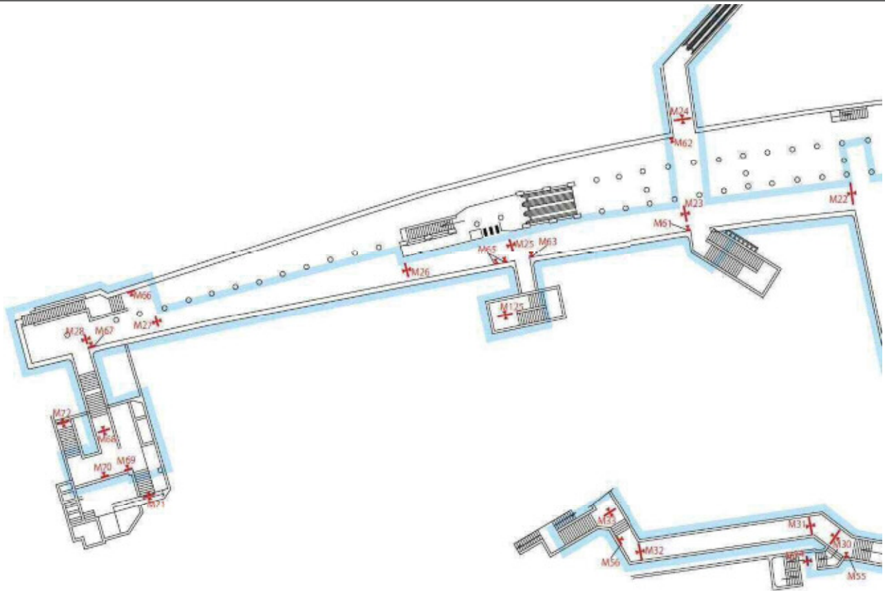
配置計画 (地下) 1/7
