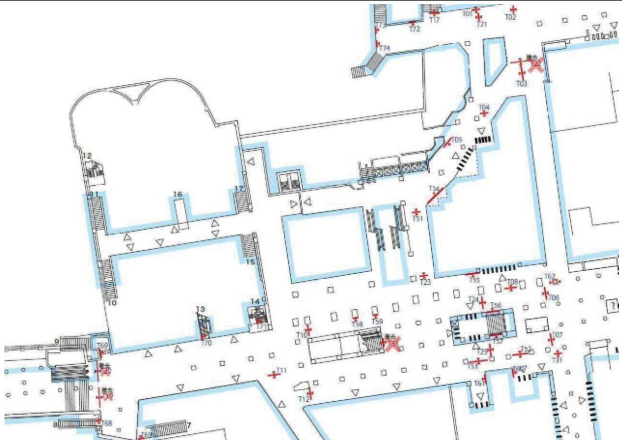
配置計画 (地下) 1/2
