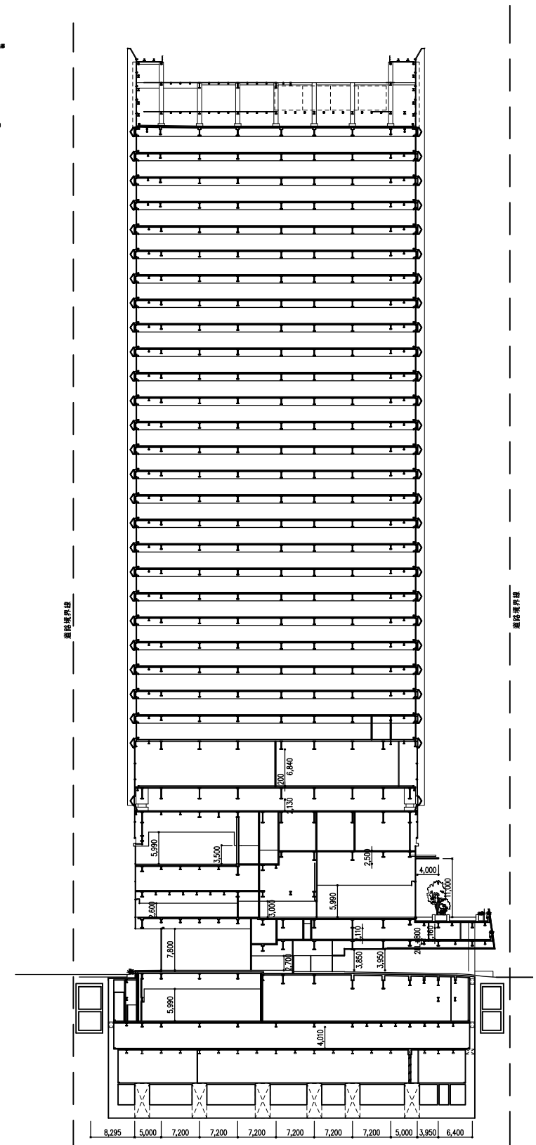
B断面図
