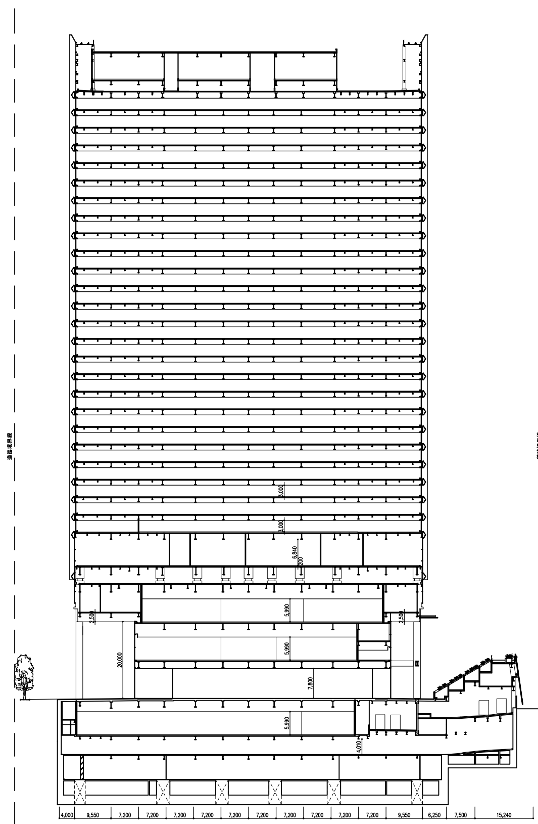
A断面図
