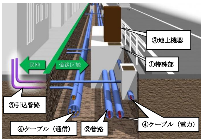
電線類をまとめて地下に収容する「電線共同溝」のイメージ
