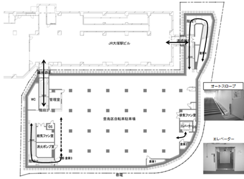
駐輪場配置図 (地下部)
