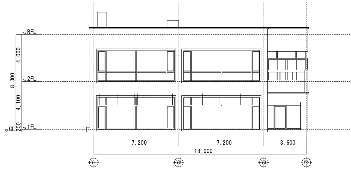
南側立面图
