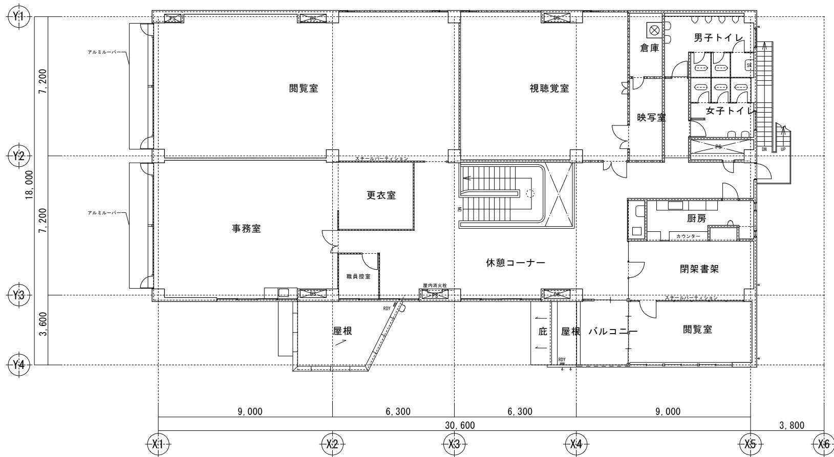
2階平面図
