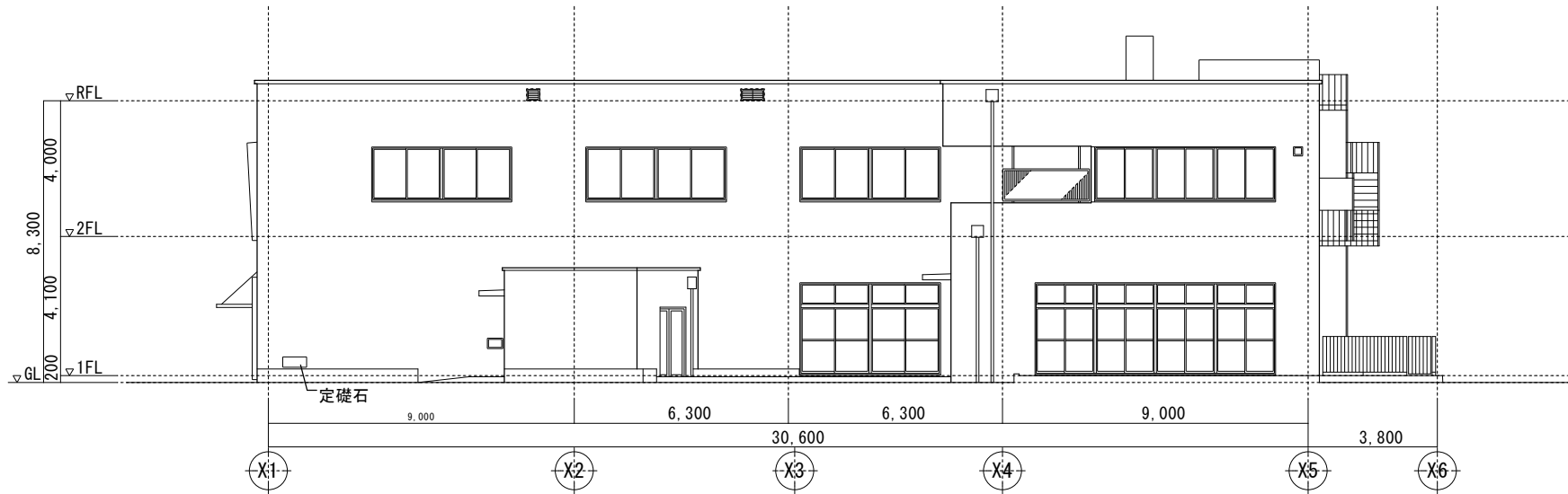
東側立面図
