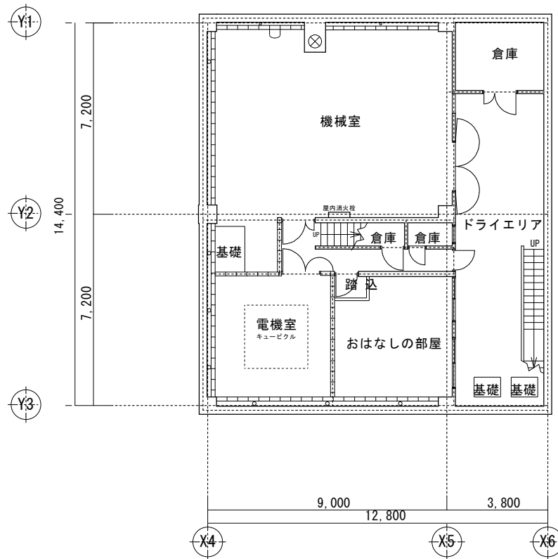
B 1 階平面図
