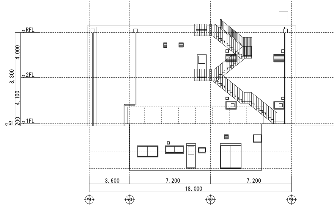
南側立面图
