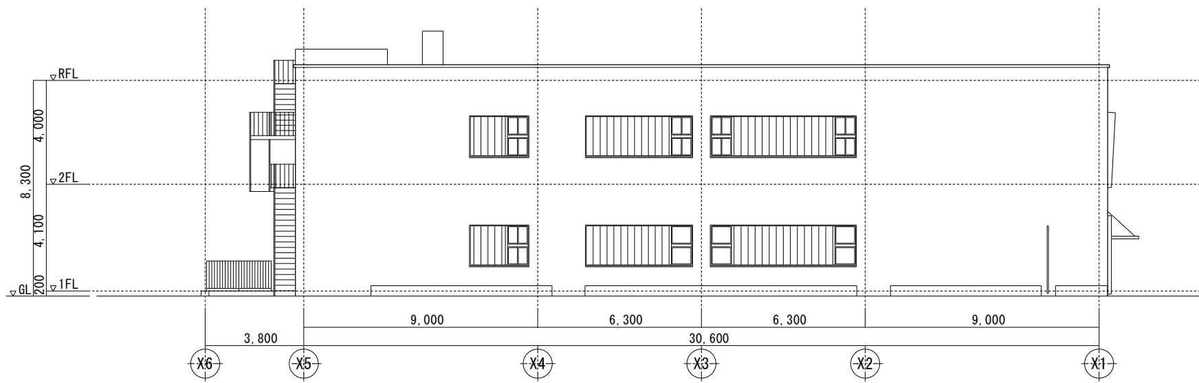
西側立面図
