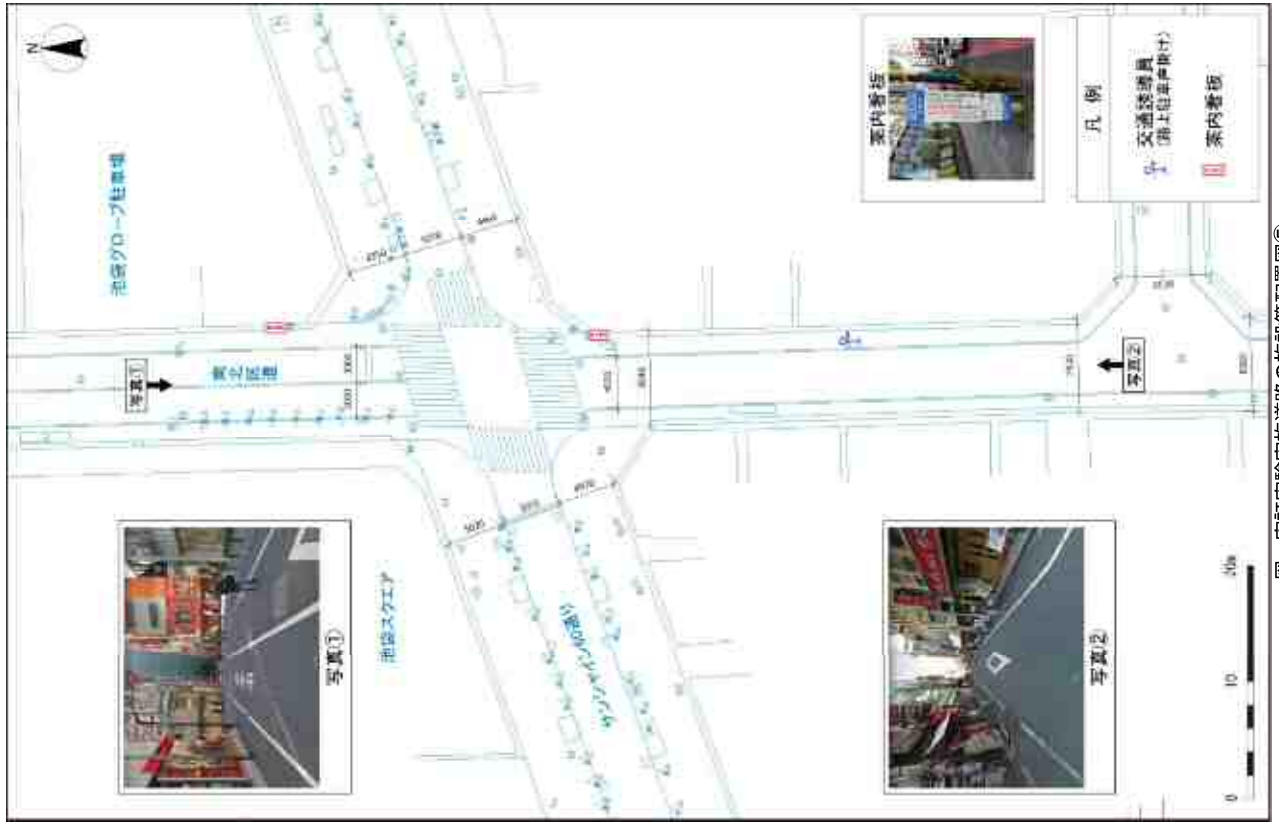
図 実証実験実施道路の施設等配置図⑤
