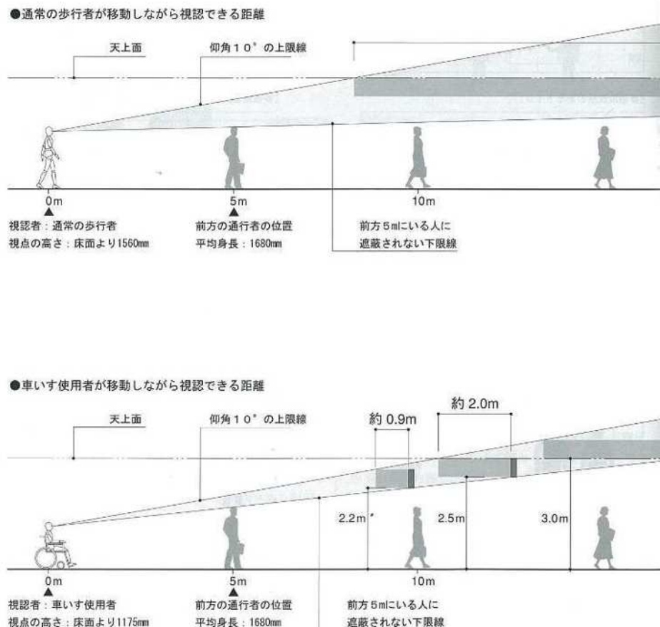
図9 視線の高さと視認できる距離
