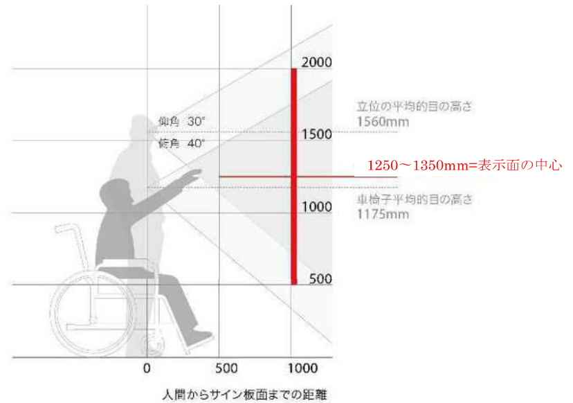
図 10 案内地図サインの高さ
